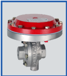
Mark 56 BPRV/66 PRV
